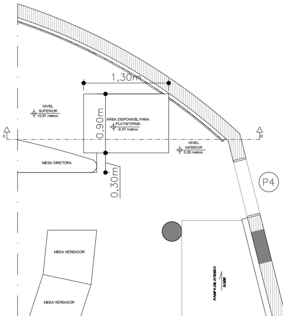
Planta baixa - Local de instalação – 2º Pavimento Plenário inferior.
