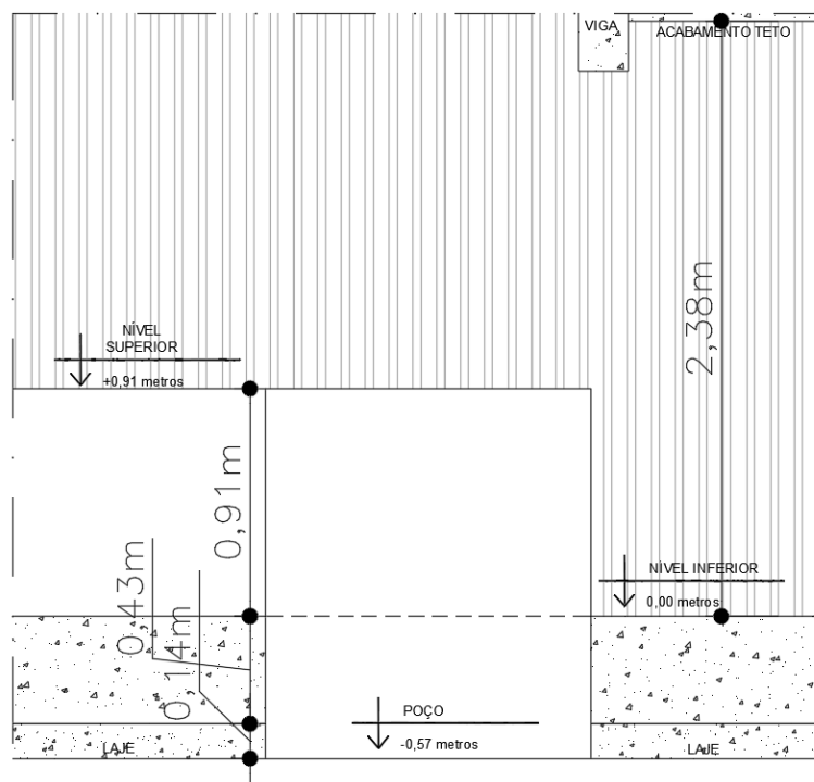
Corte Esquemático - Local de instalação – 2º Pavimento Plenário inferior.
