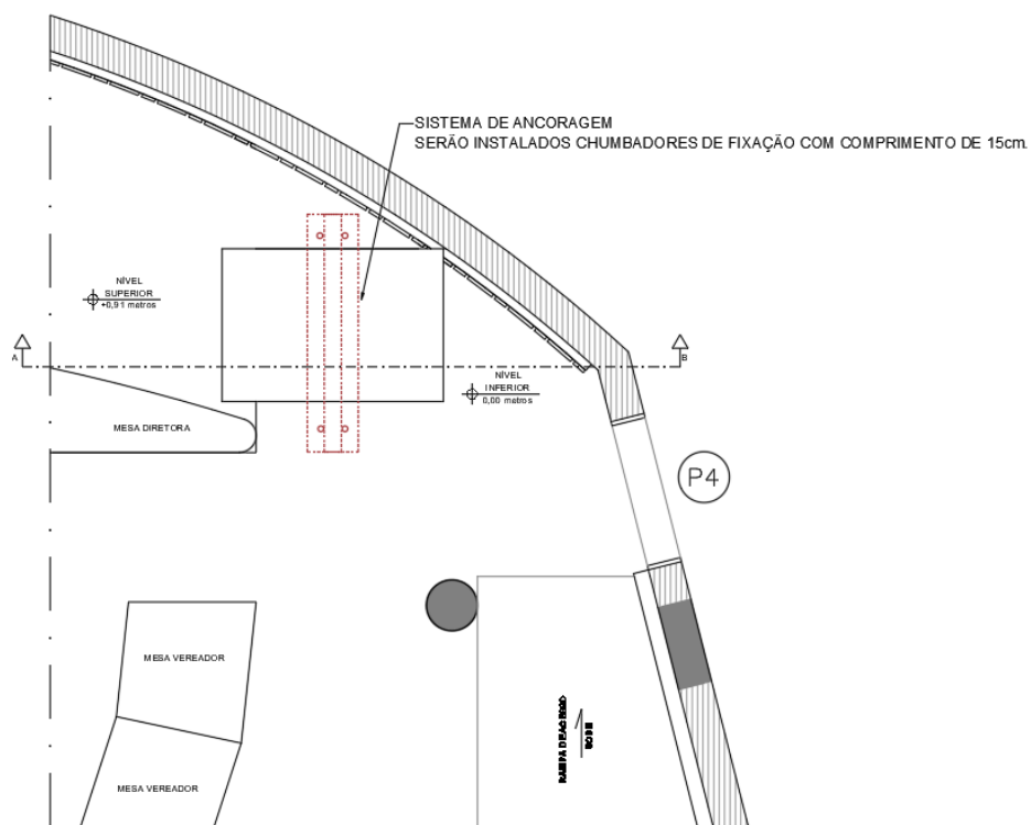
Demarcação do Sistema de Ancoragem – 1º Pavimento Garagem
